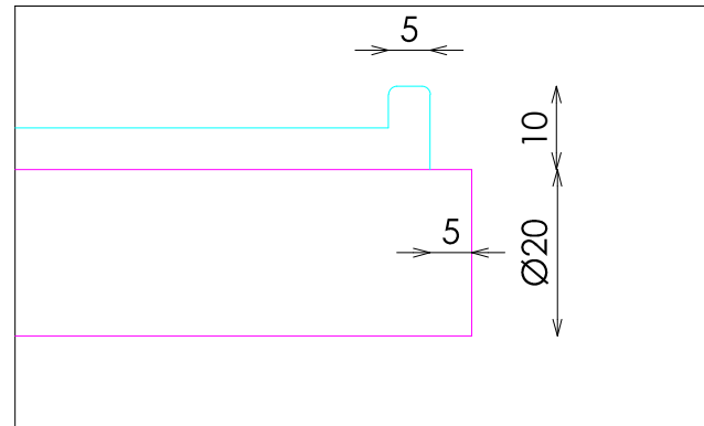
DETALLE ANTIROCE
