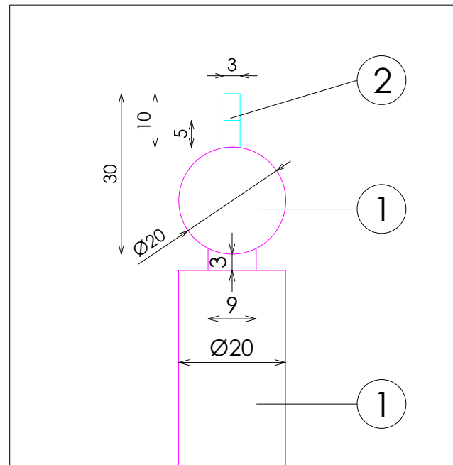
DETALLE ANTIROCE
