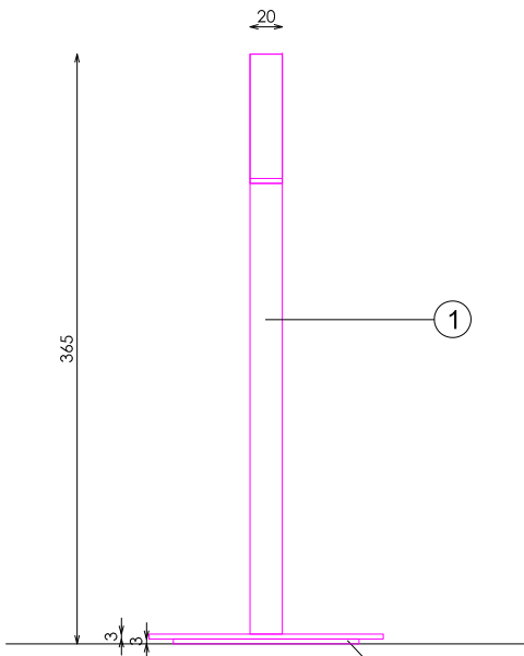
ALZADO
