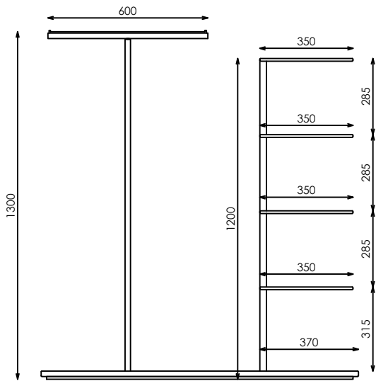
ALZADO
