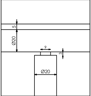
DETALLE C
