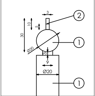
DETALLE ANTIROCE
