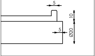
DETALLE ANTIROCE
