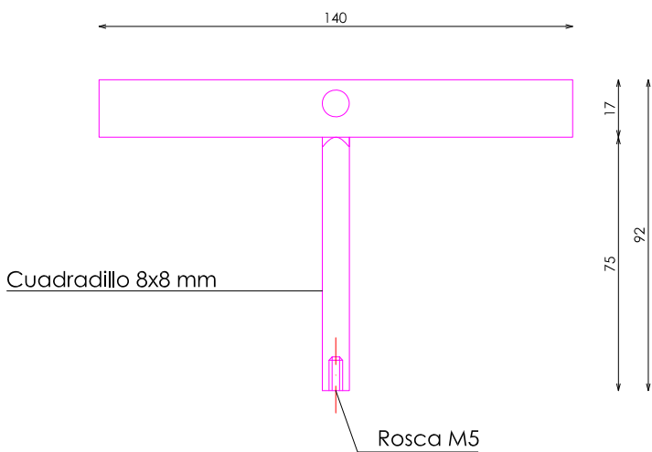
ALZADO
