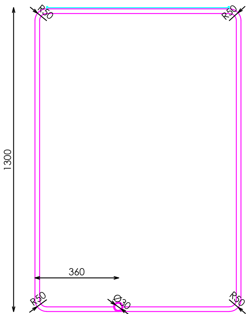
ALZADO
