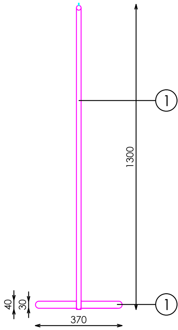
PERFIL
