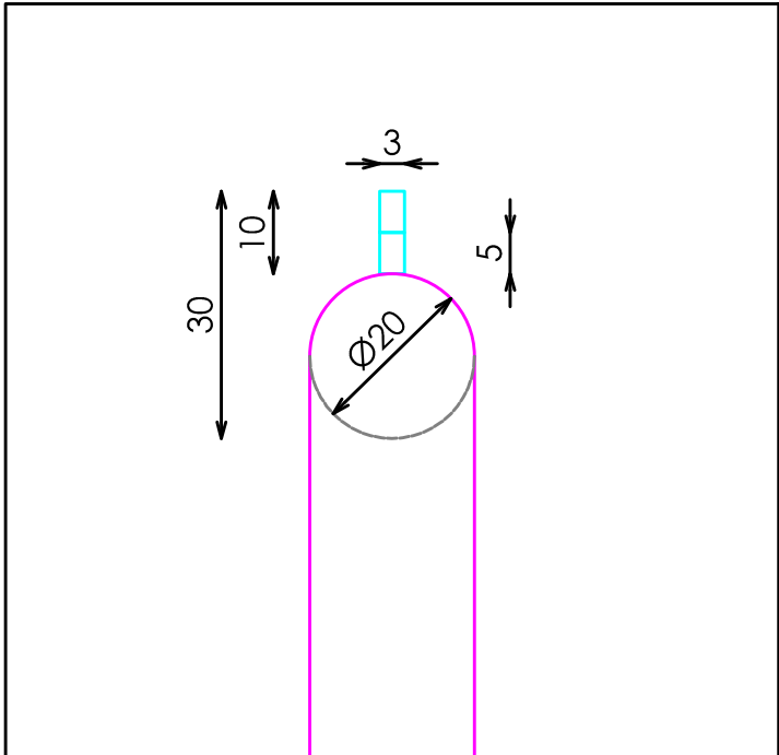
DETALLE A
