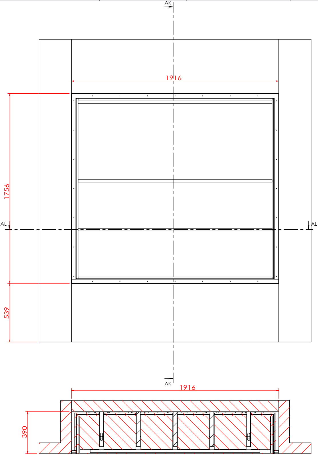
剖面 AL-AL
