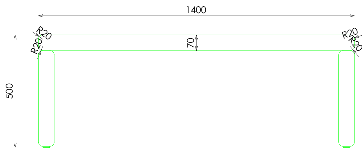
ALZADO
