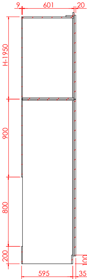
剖面 AG-AG
