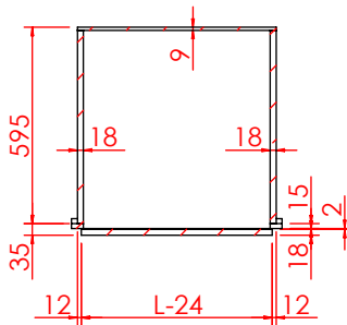
剖面 AH-AH
