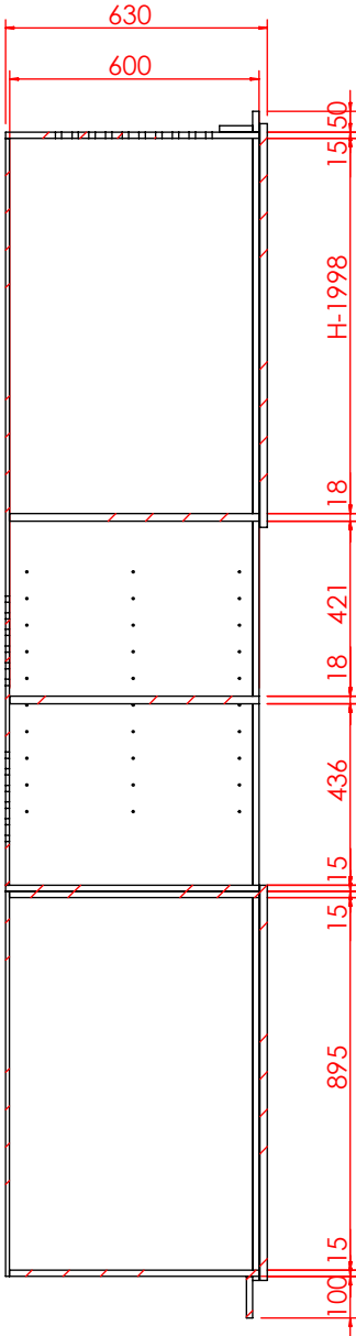
剖面 AG-AG
