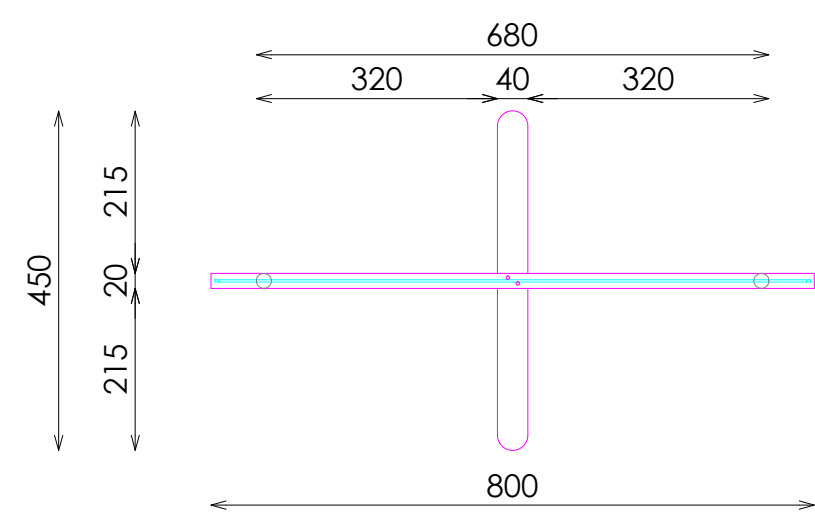
PLANTA
