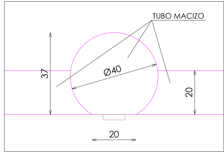
DETALLE D
