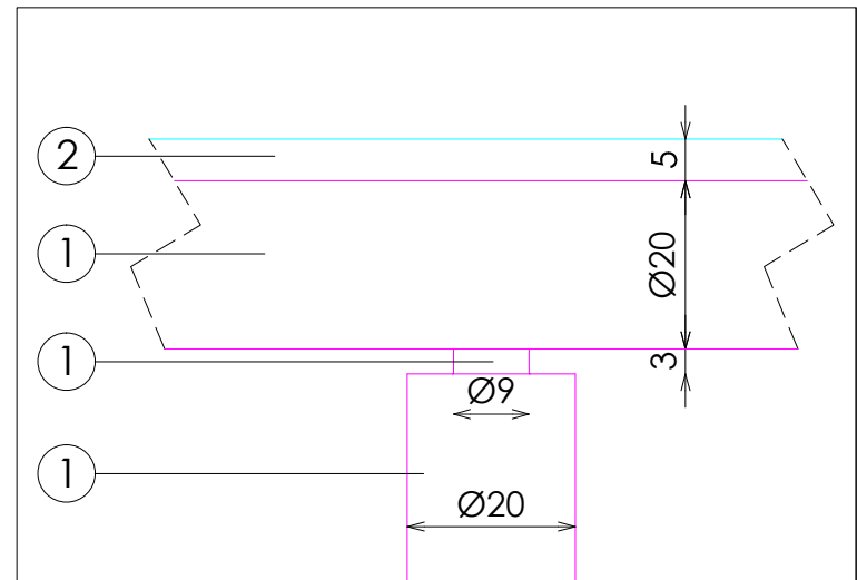
DETALLE B
