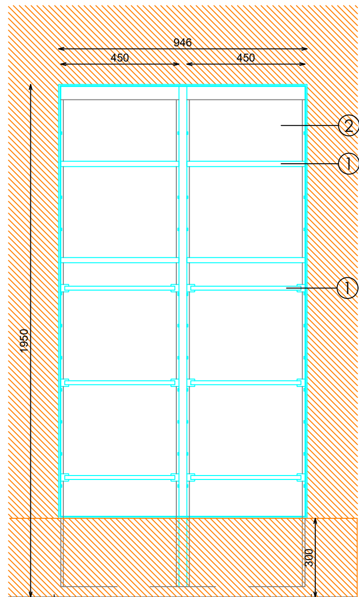
ALZADO
