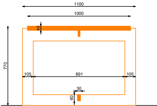
SECCION LATERAL
