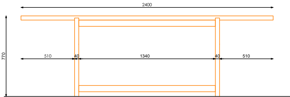
ALZADO FRONTAL
