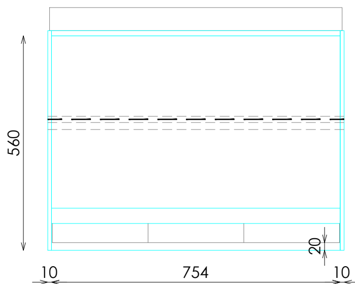
PLANTA PANTALLA
