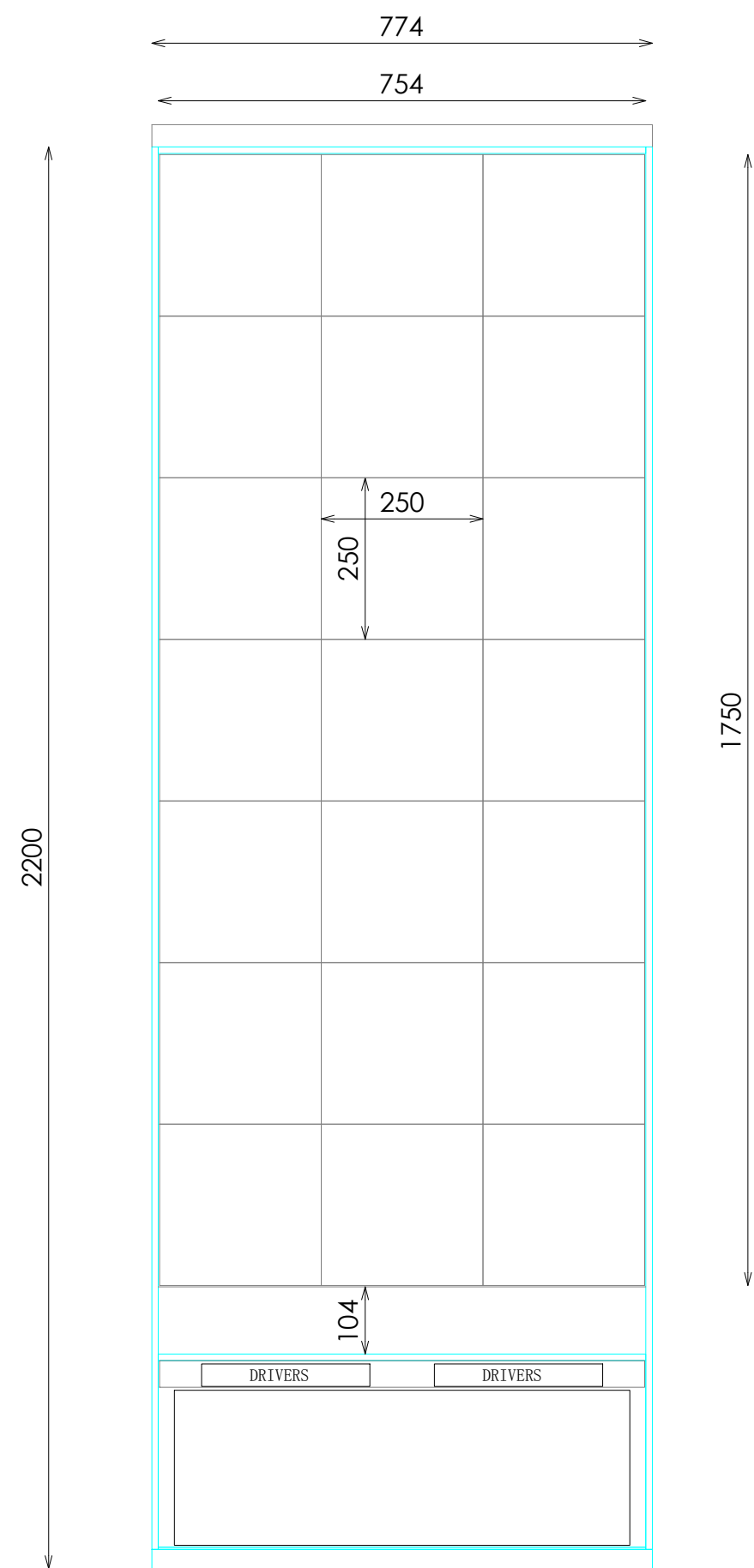
ALZADO
