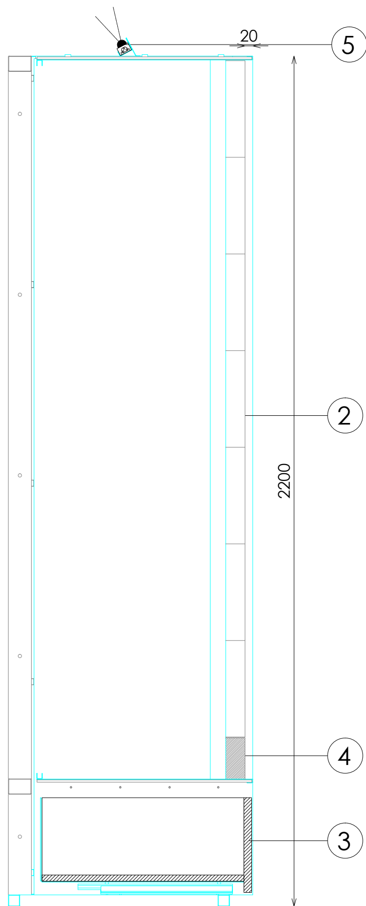
SECCIÓN
