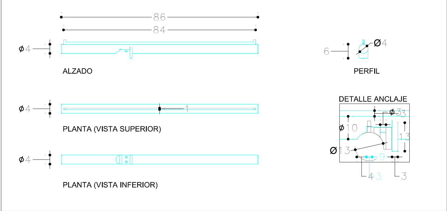
DETALLE FRONTALES EXTRAIBLES
