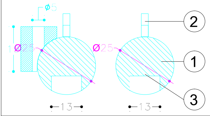
DETALLE BARRA
