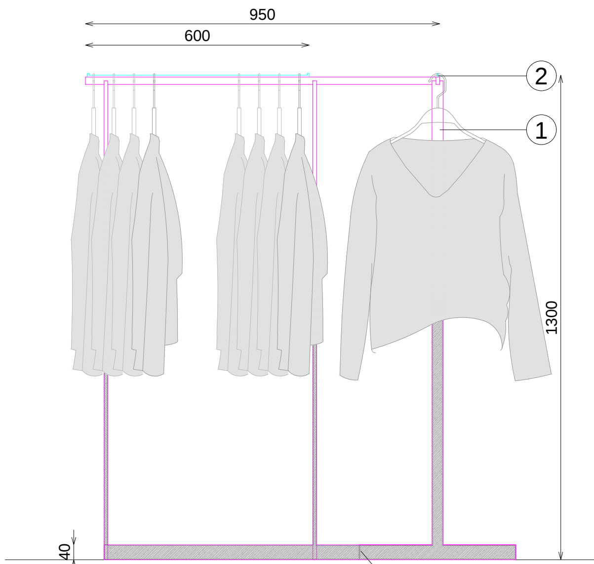
ALZADO LATERAL
