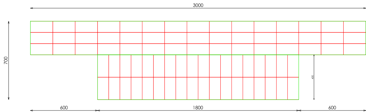
ALZADO
