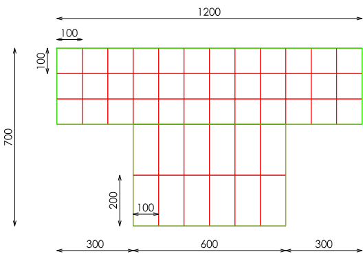
PERFIL
