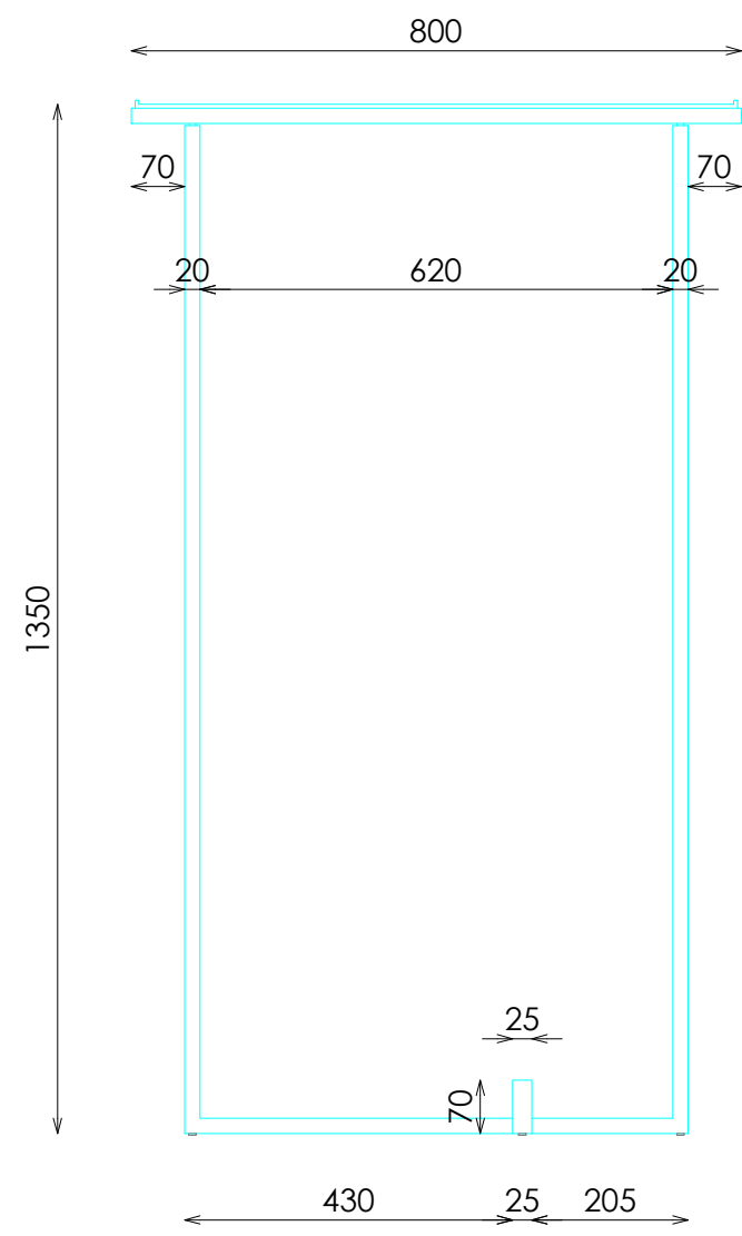
ALZADO
