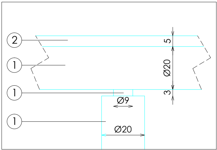
DETALLE B
