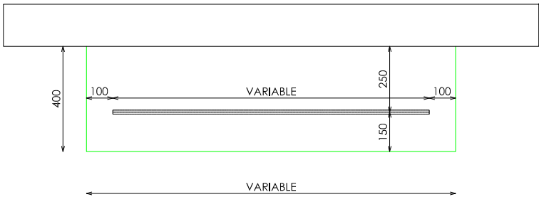
PLANTA
