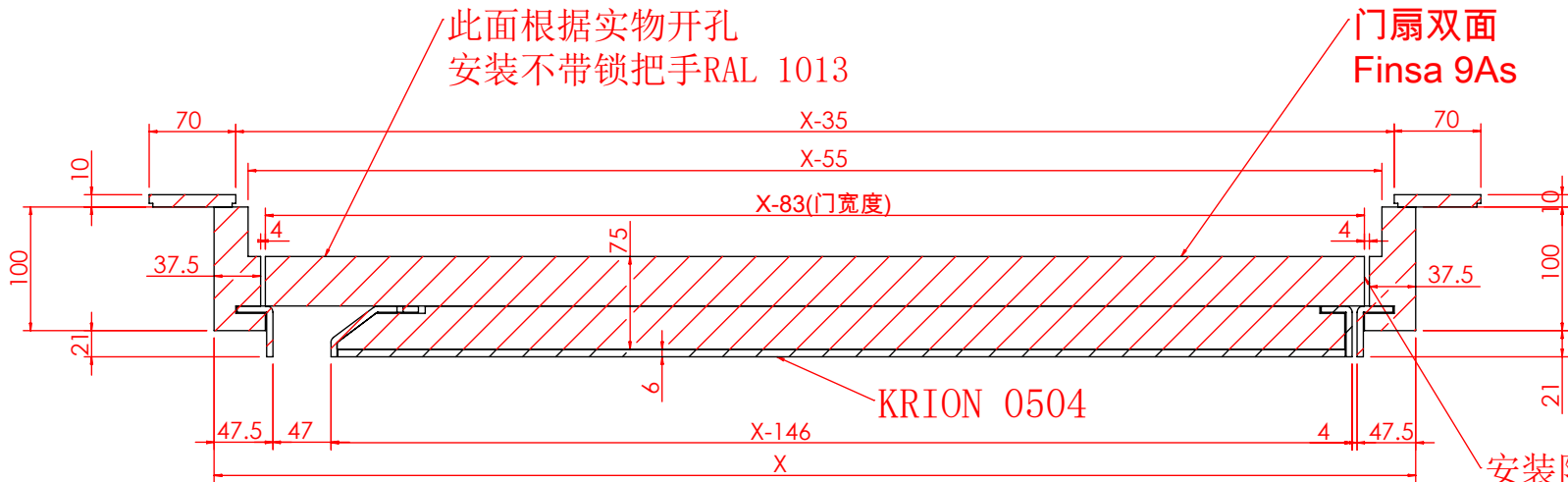
剖面 AH-AH 比例 1:6
