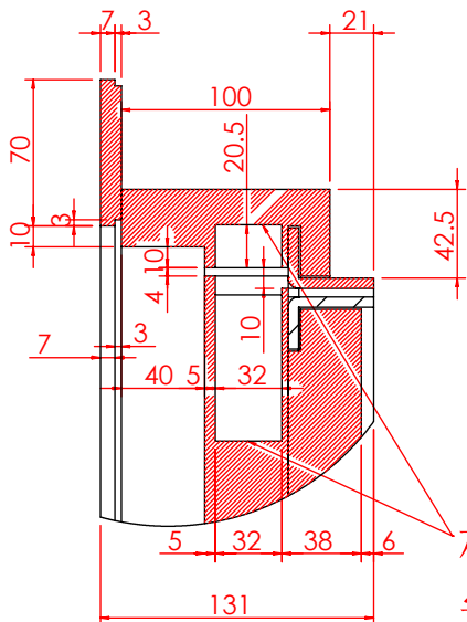
局部视图 AI 比例 1:4
