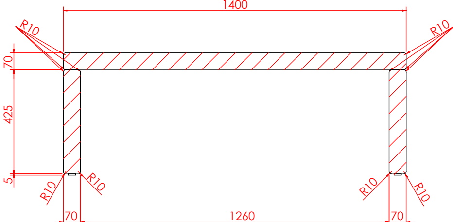
剖面 AG-AG
