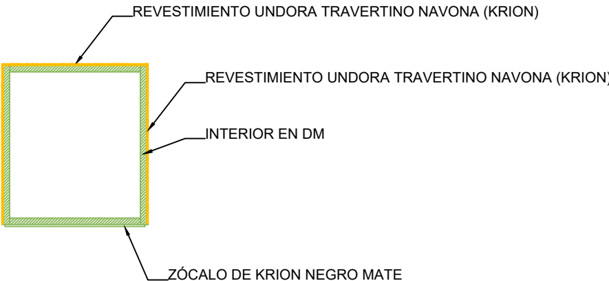
SECCIÓN SECTION
