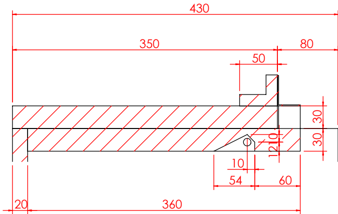
局部视图 AJ 比例 1 : 5
