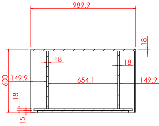
剖面 AN-AN
