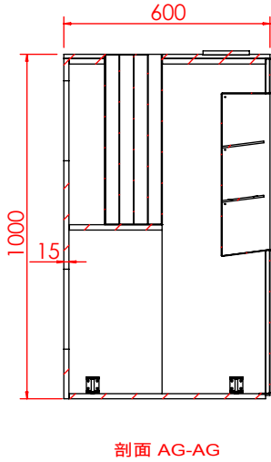
剖面 AG-AG
