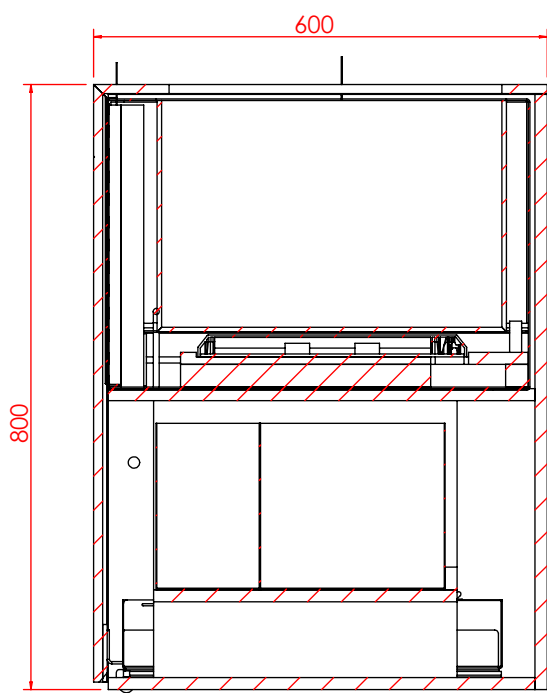
剖面 AH-AH 比例 1 : 10
