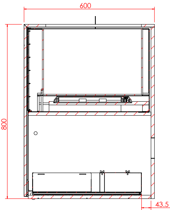
剖面 AG-AG 比例 1 : 10
