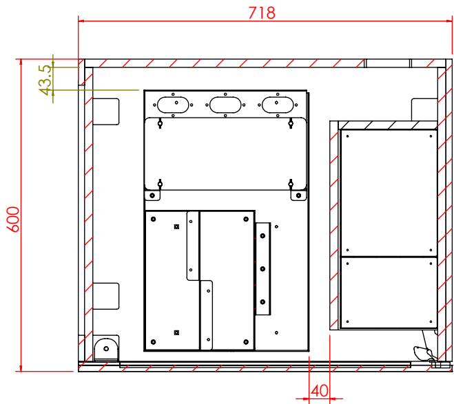
剖面 AI-AI 比例 1 : 10
