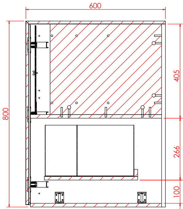
剖面 AG-AG 比例 1 : 10
