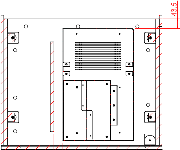
剖面 AI-AI 比例 1 : 10
