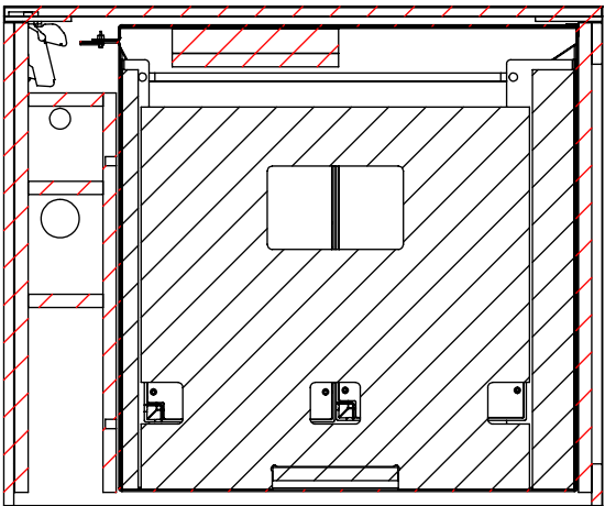
剖面 AI-AI 比例 1 : 10
