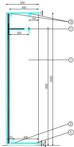
SECCIÓN
