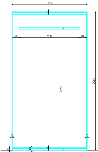
ALZADO
