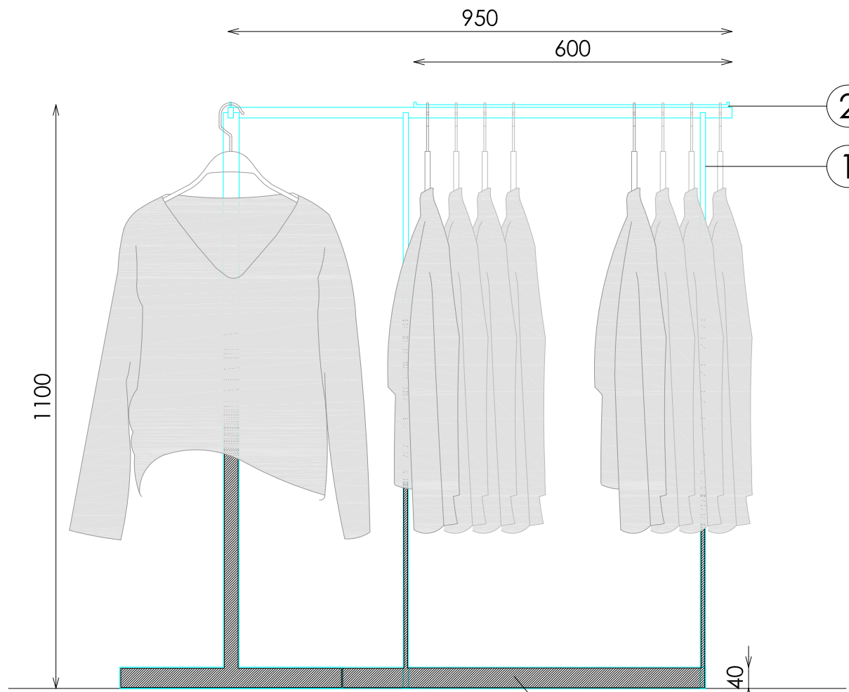
ALZADO LATERAL
