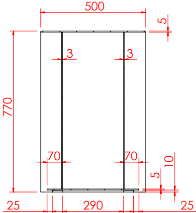
剖面 AH-AH
