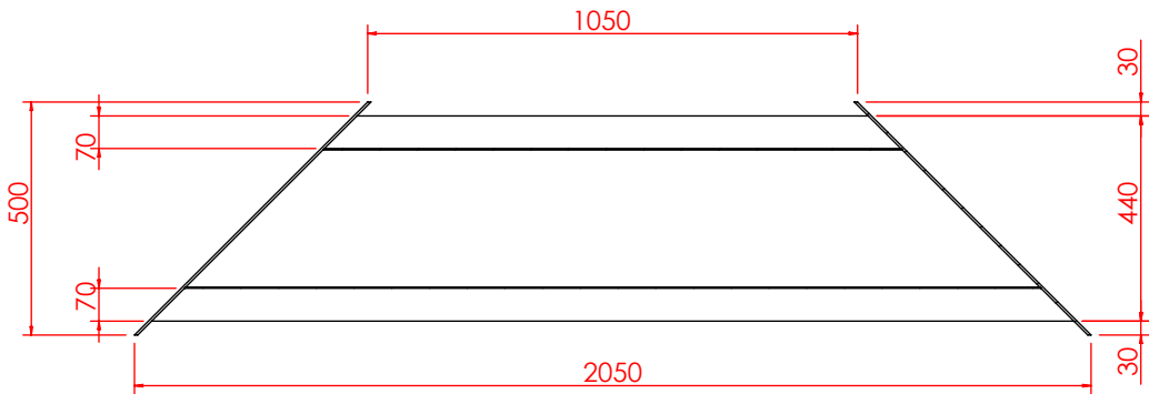
剖面 AG-AG
