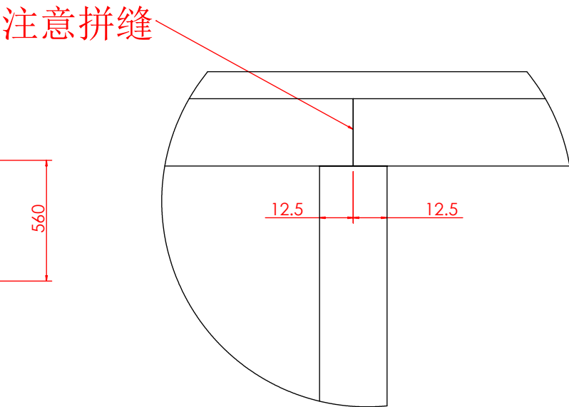
局部视图 AG 比例 1 : 2
