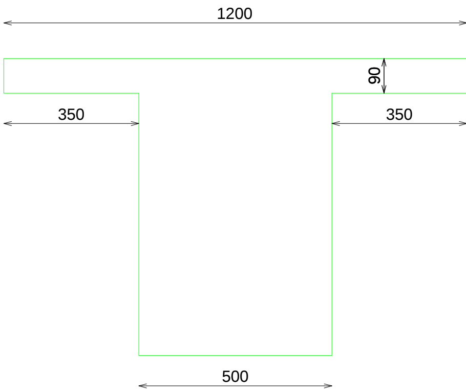
ALZADO LATERAL
