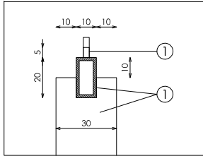
DETALLE B
