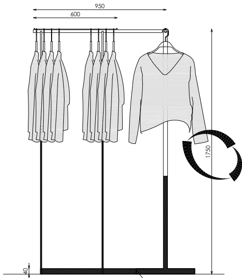
ALZADO LATERAL
