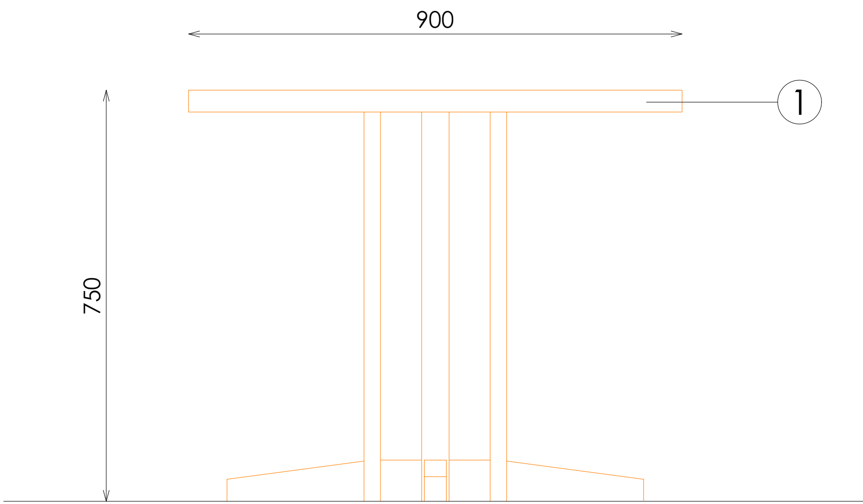
ALZADO LATERAL
