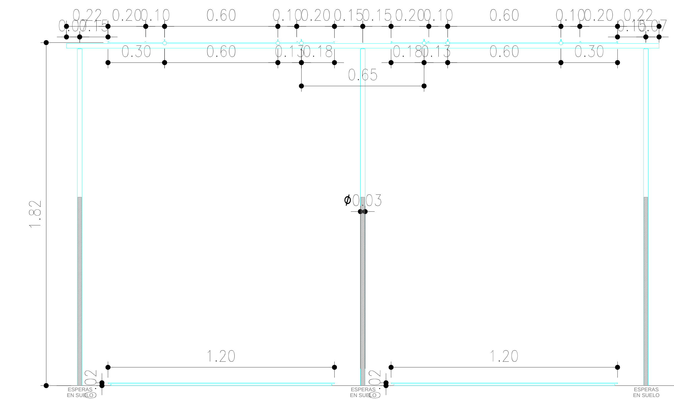
ALZADO FRONTAL
