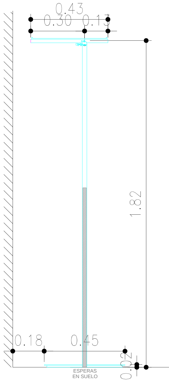
SECCIÓN
