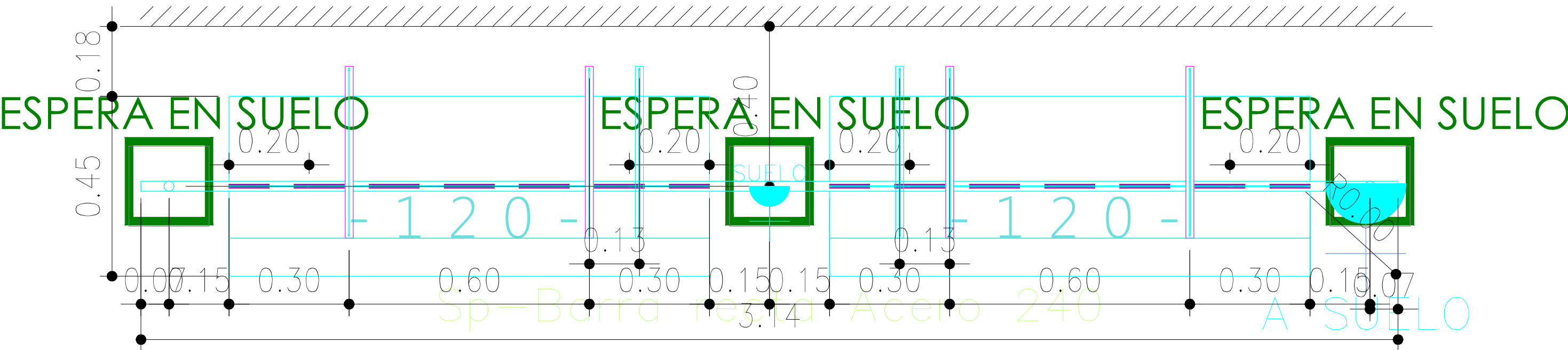
PLANTA
