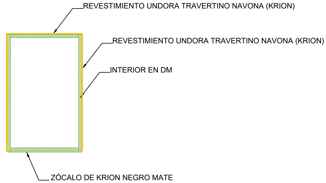
SECCIÓN SECTION
