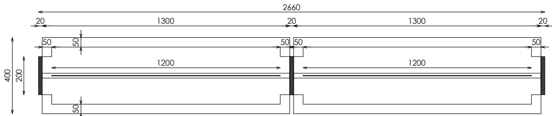
PLANTA SECCIONADA
