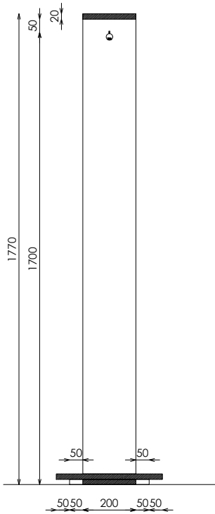
SECCIÓN
