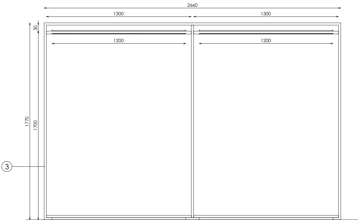
ALZADO
