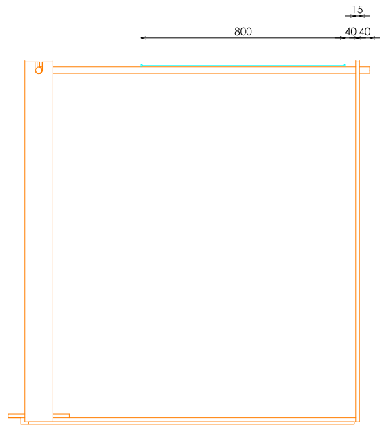
ALZADO
