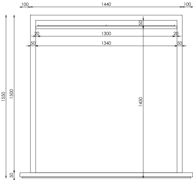
ALZADO
