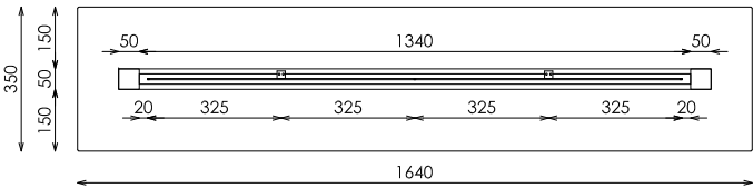
PLANTA SECCIONADA
