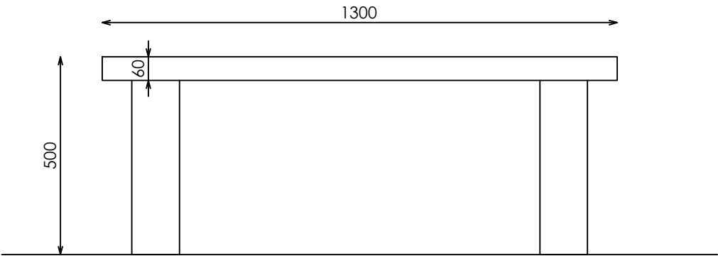
ALZADO
