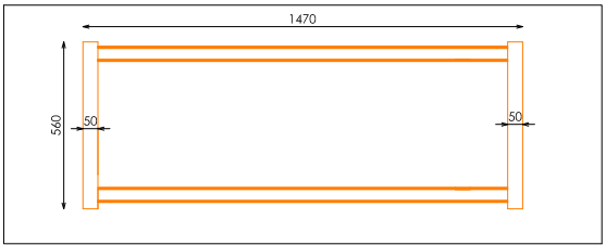
PLANTA (PATAS)
