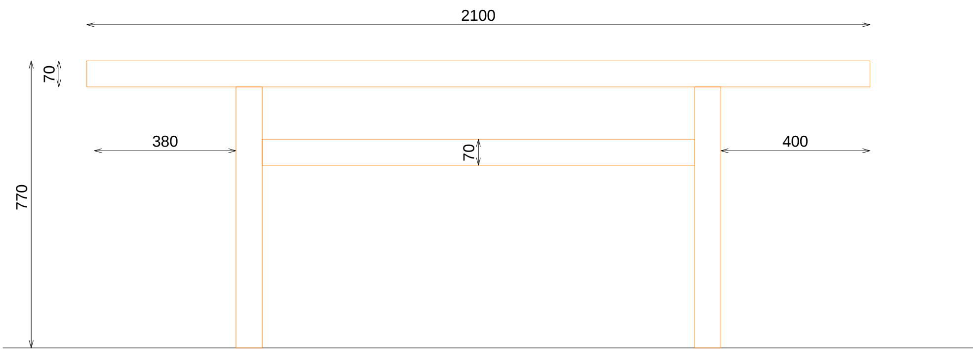
ALZADO FRONTAL
