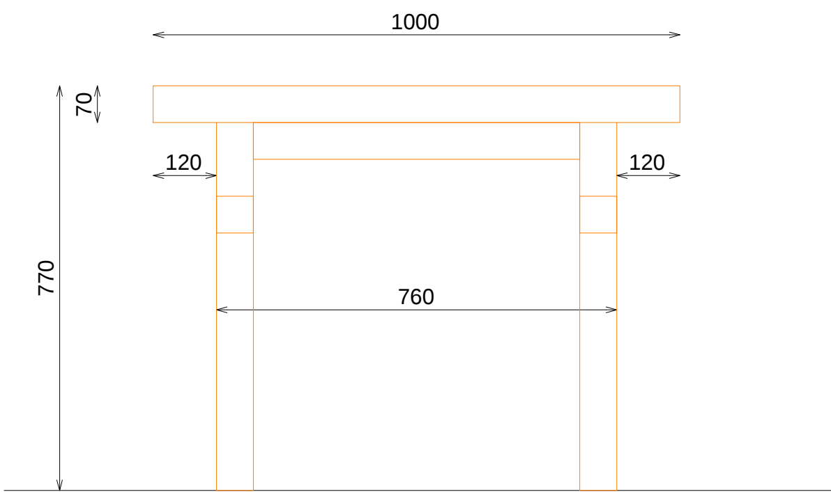
ALZADO LATERAL
