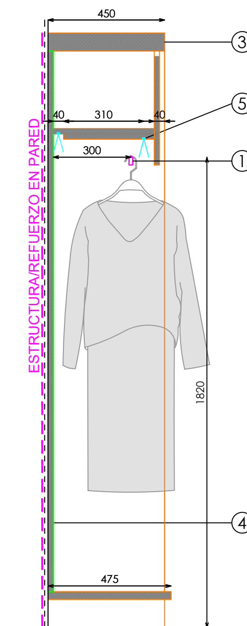
SECCIÓN BARRA ALTA
