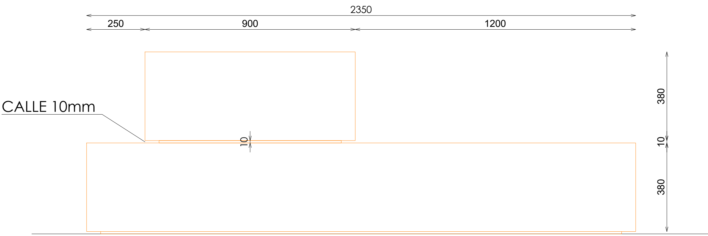
ALZADO LATERAL
