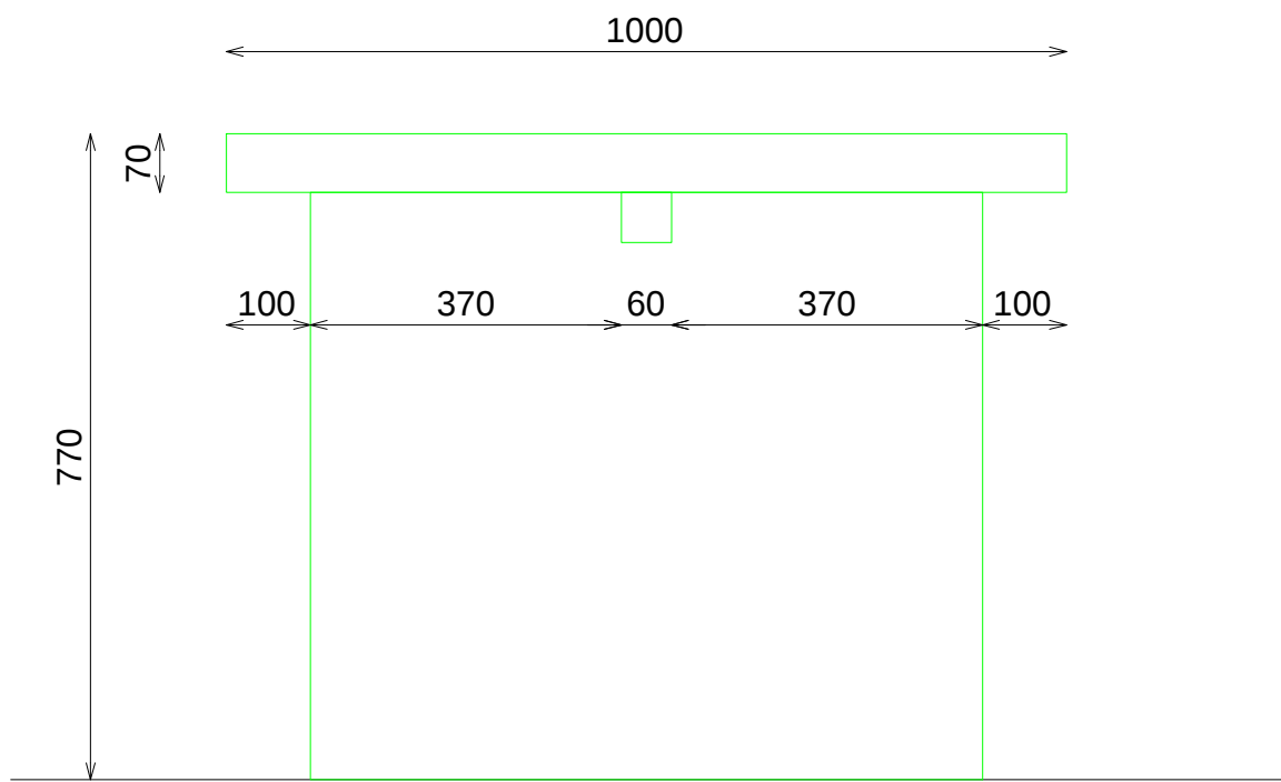
SECCION LATERAL
