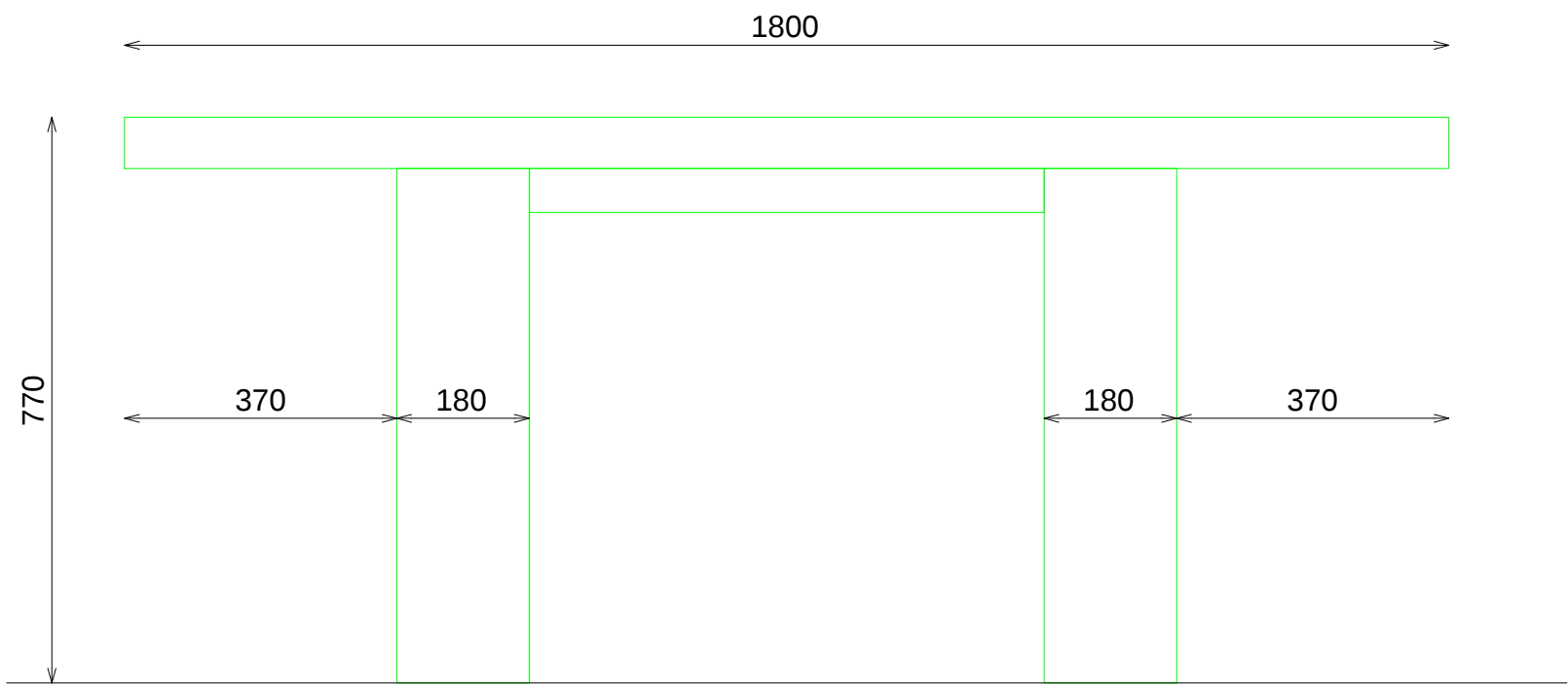
ALZADO FRONTAL
