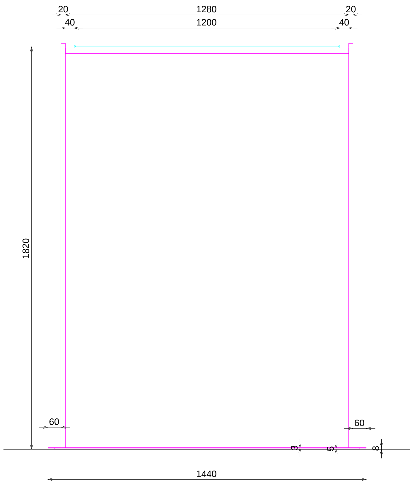
ALZADO SECCIONADO
