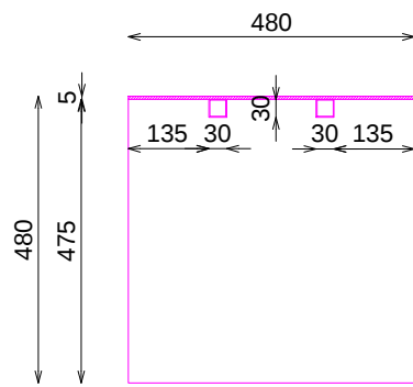
SECCIÓN
