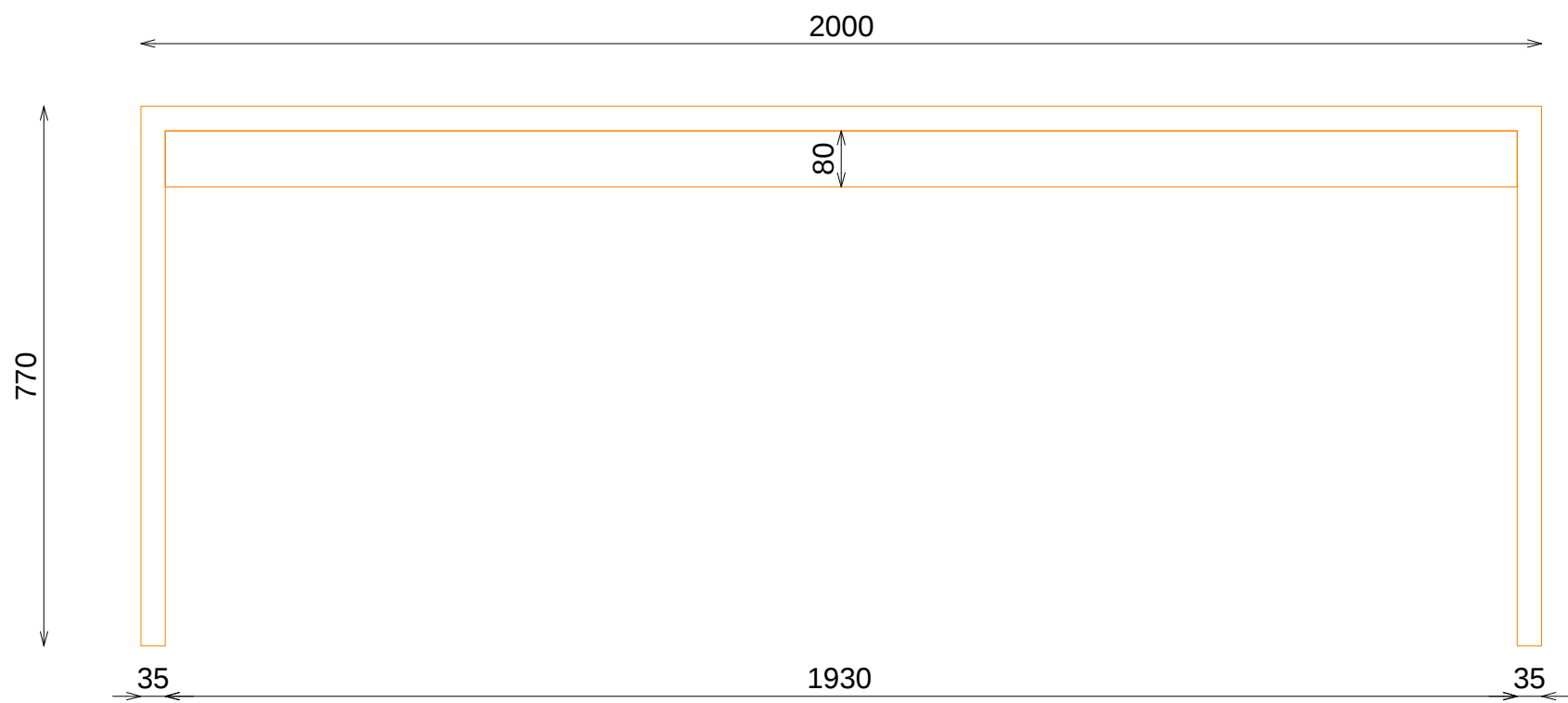
ALZADO FRONTAL
