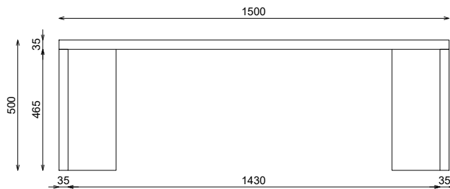
ALZADO POSTERIOR
