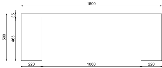
ALZADO FRONTAL
