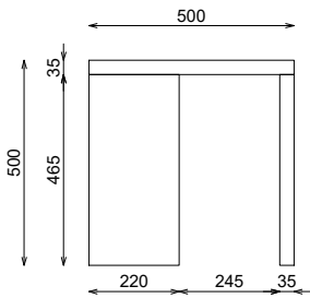
ALZADO LATERAL
