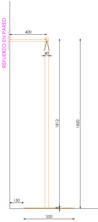
PERFIL SECCIONADO
