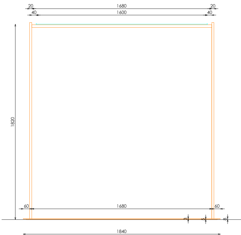
ALZADO SECCIONADO
